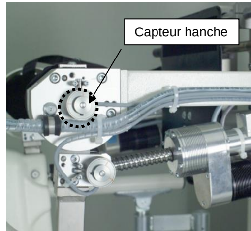
Figure 17 : Capteur angulaire
