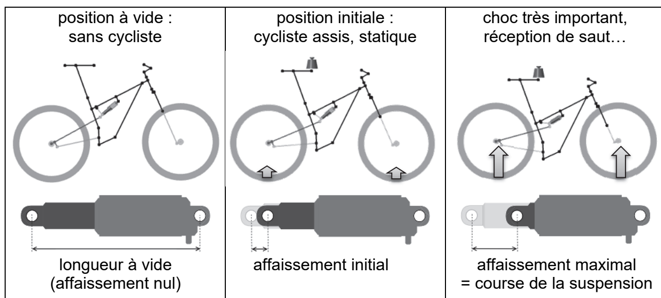
Figure 2 : affaissements aux positions remarquables de la suspension
