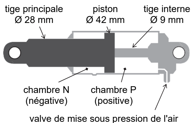
Figure 8 : ressort pneumatique
