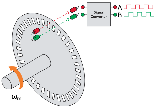
Figure 14 : codeur incrémental
