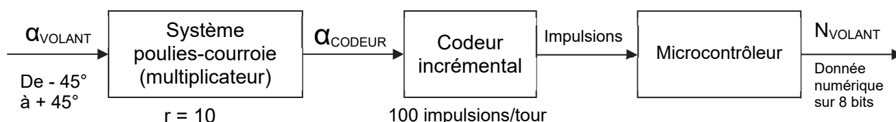
Figure 13 : chaîne d'acquisition de l'angle volant
